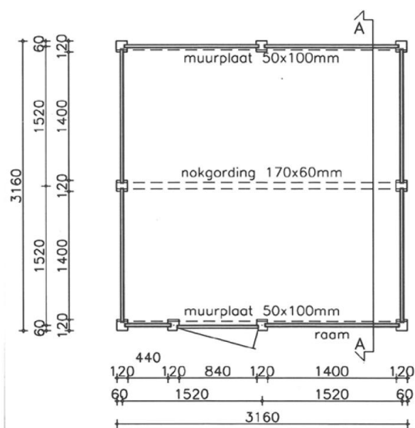
PLATTEGROND
